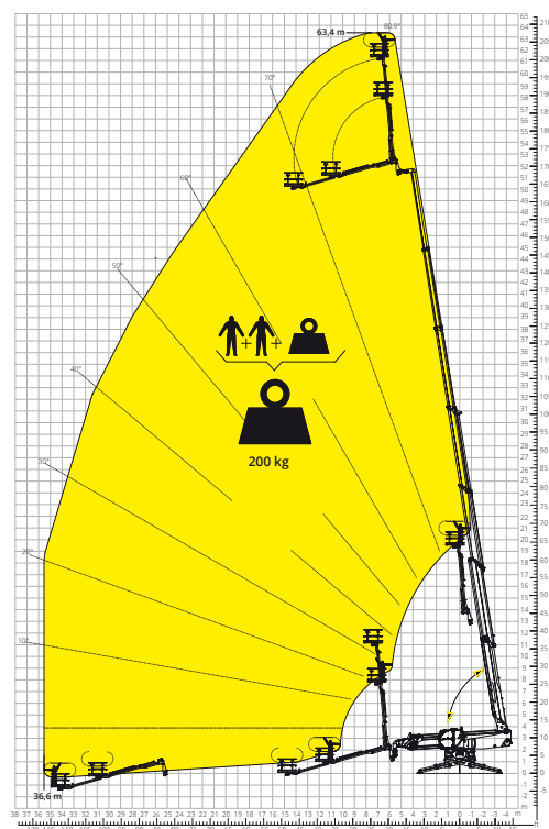
Lastdiagramm mit TELESKOPARBEITSKORB 200 kg - 10 m ATT - 01 - 022
