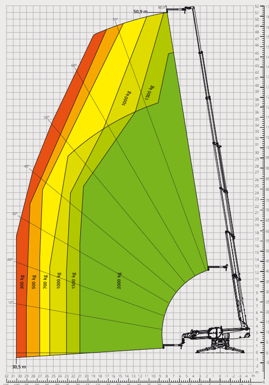
Lastdiagramm mit AUSLEGER 2.000 kg ATT-04-013
