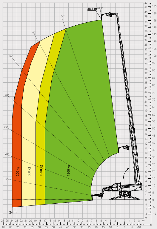
Lastdiagramm mit AUSLEGER MIT SEILWINDE 1.500 kg ATT - 04 - 011
