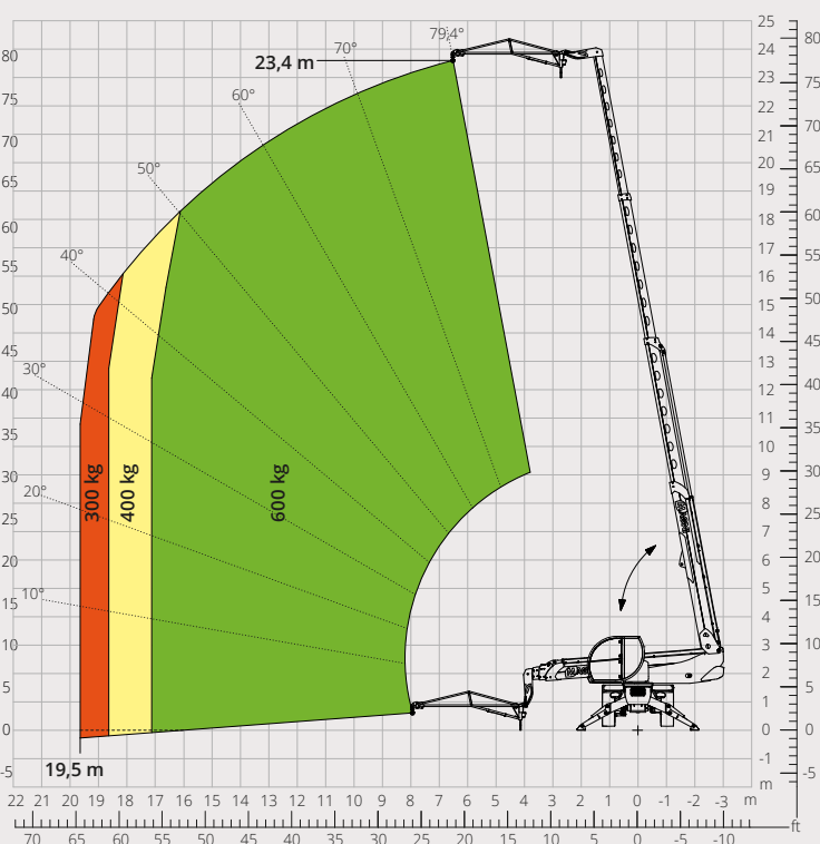
Diagramma portate con BRACCETTO SCATOLATO 600 kg ATT - 04 - 001
