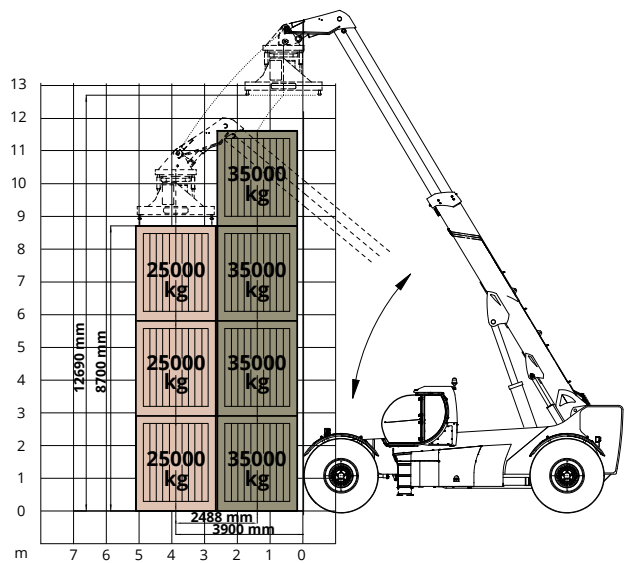
Lastdiagram met vorken voor containers 20"-40"
